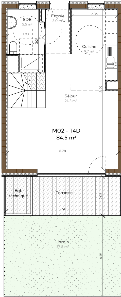
Plan RDC
